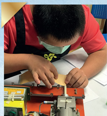
將紙條放上輔具「筆蓋形單手捲紙機」。
